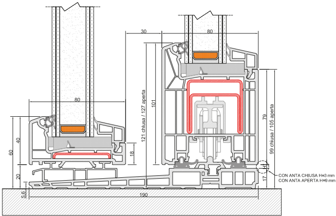
Nodo Inferiore Anta panoramica
