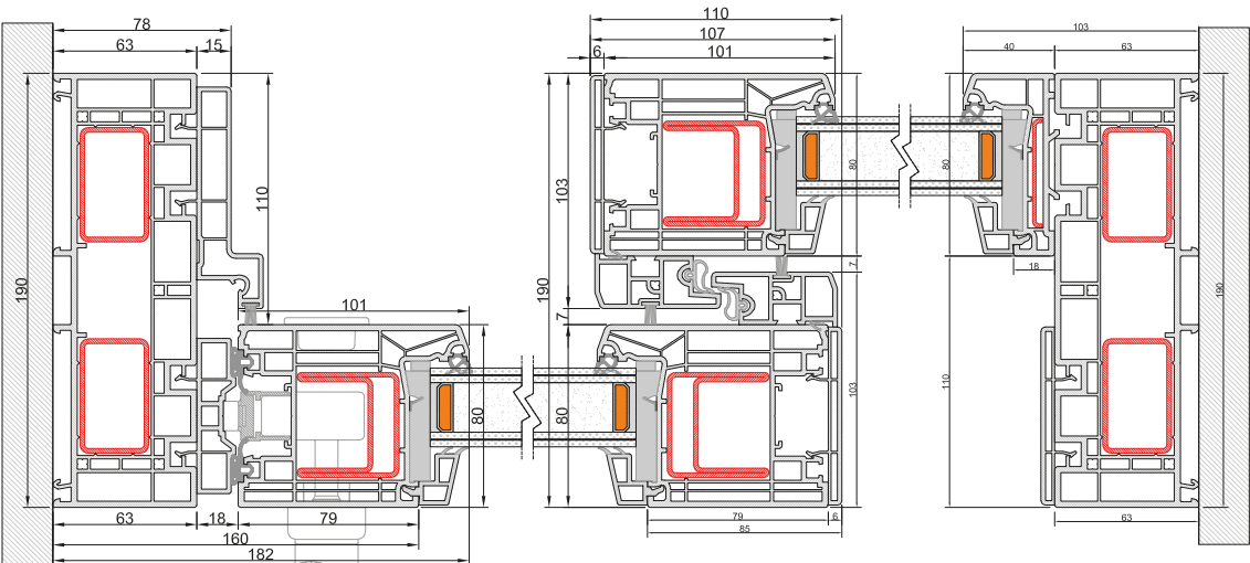
Nodo Centrale Anta panoramica
